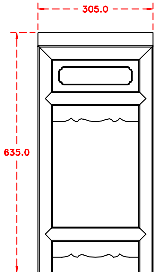
End Elevation
